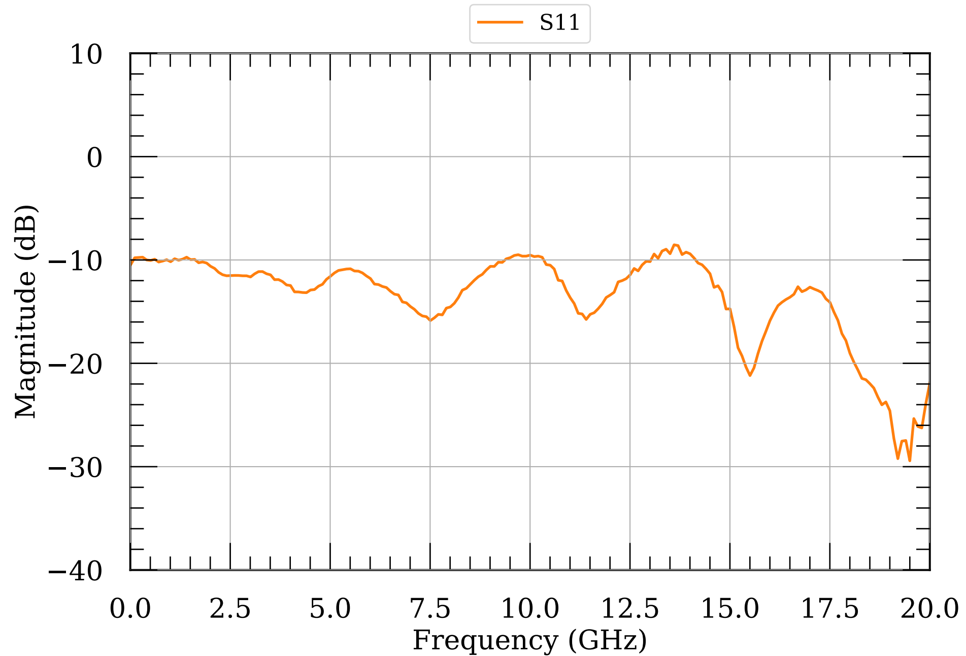
LNA S-params module027v2
